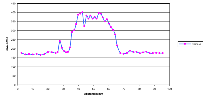
Vickershärte Probe M7
