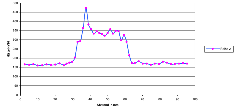
Vickershärte Probe M7
