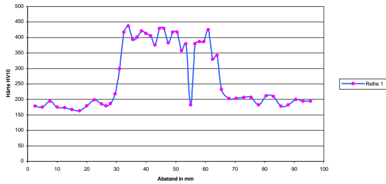
Vickershärte Probe M7
